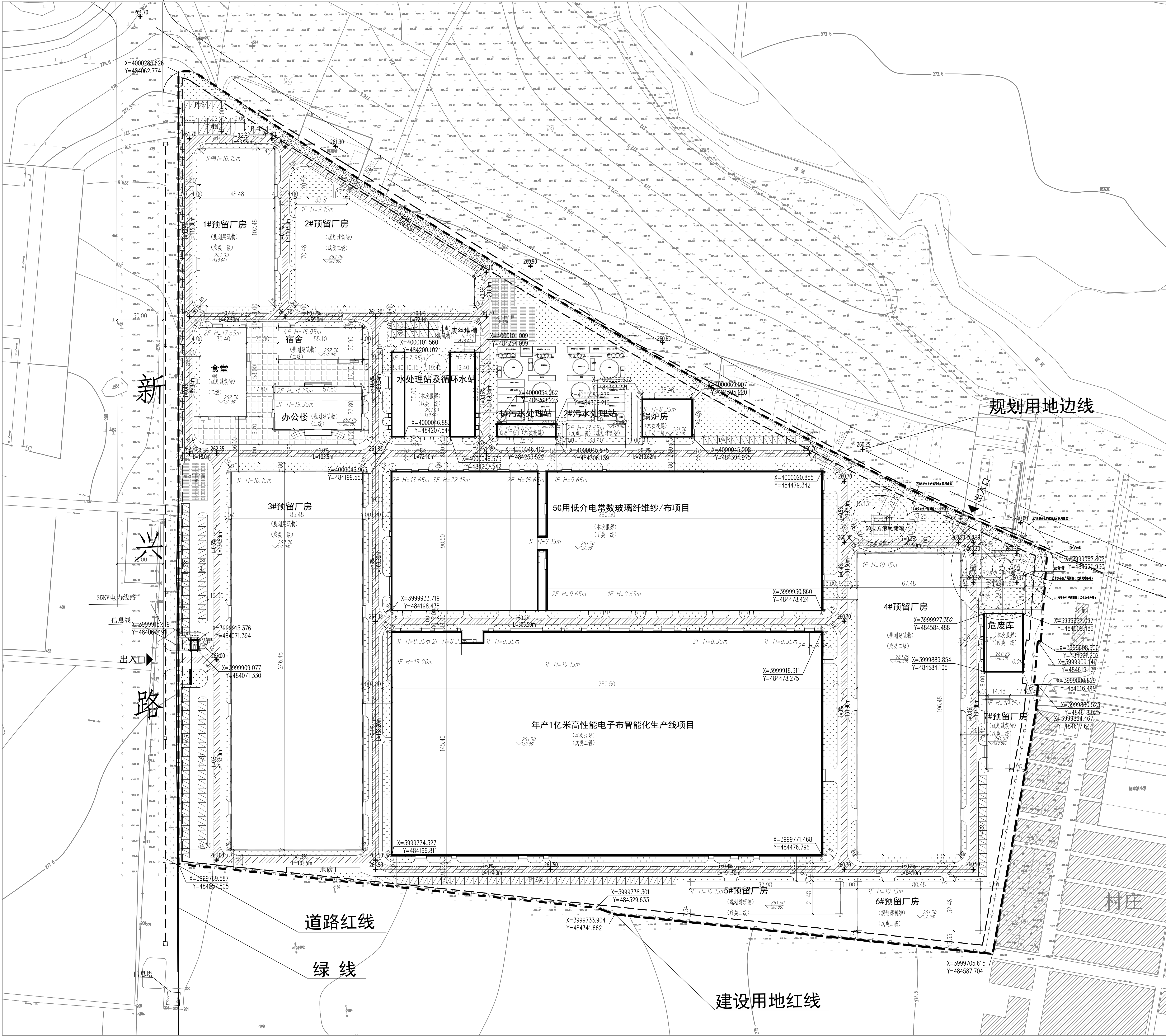
总平面图 1:1000
